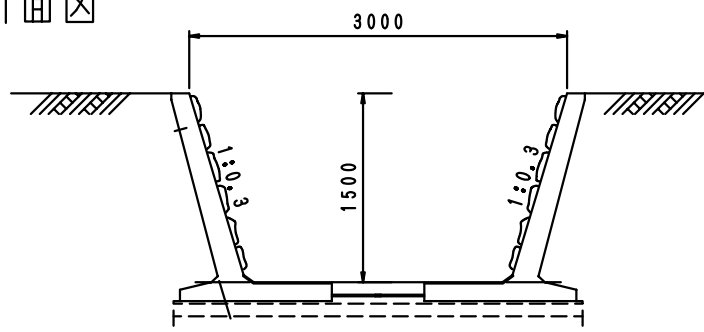
施工断面図
