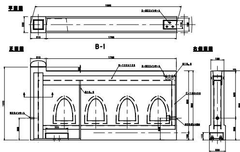
車道基本構造図 1/100
