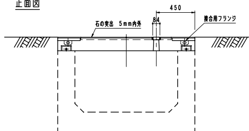
正面図
