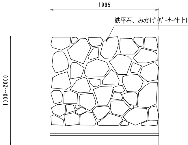
正面図
